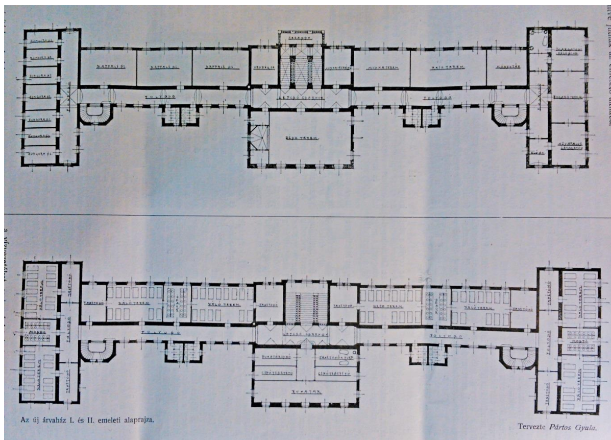
Alaprajz, első és második emelet, fotó: Építő Ipar, 26. szám, 1907. június 7., 264. o.
